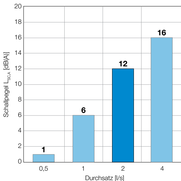
Schallpegel L_{SC,A} Triplus® gemäß EN 14366
