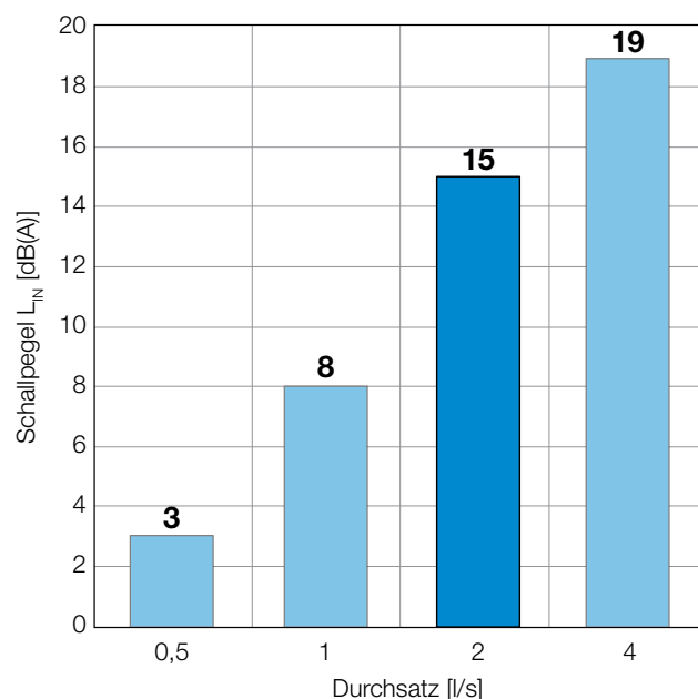
Schallpegel L_{IN} Triplus® gemäß DIN 4109
