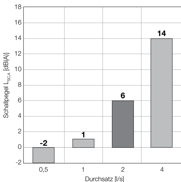
Schallpegel L_{SC,A} Silere® gemäß EN 14366
