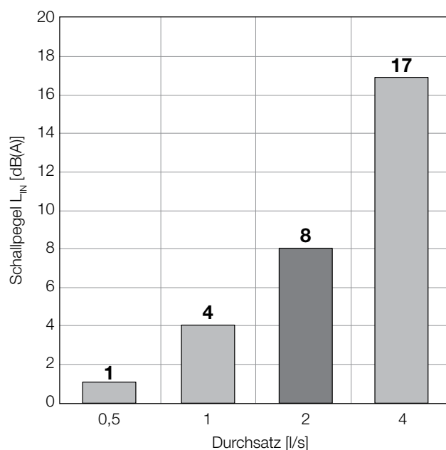
Schallpegel L_{IN} Silere® gemäß DIN 4109
